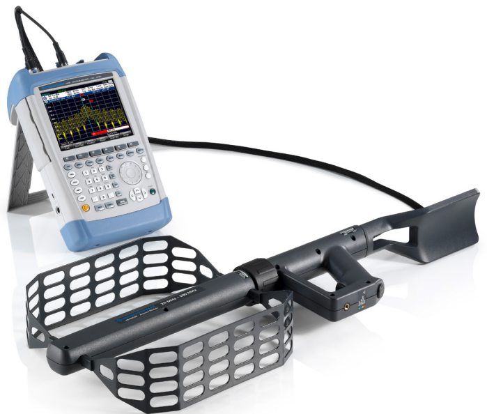
R&S®FSHとR&S®HE400 アンテナ
