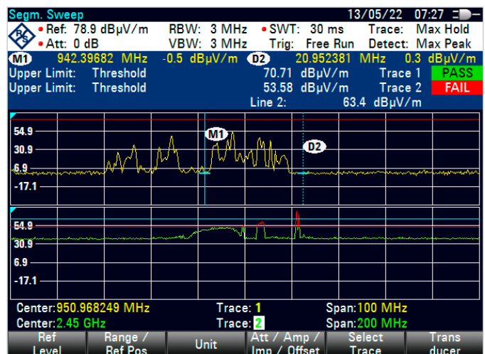
R&S®FSH-K20 セグメント掃引オプション
