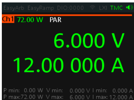
Paralleler Betrieb
