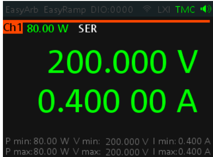
Serieller Betrieb
