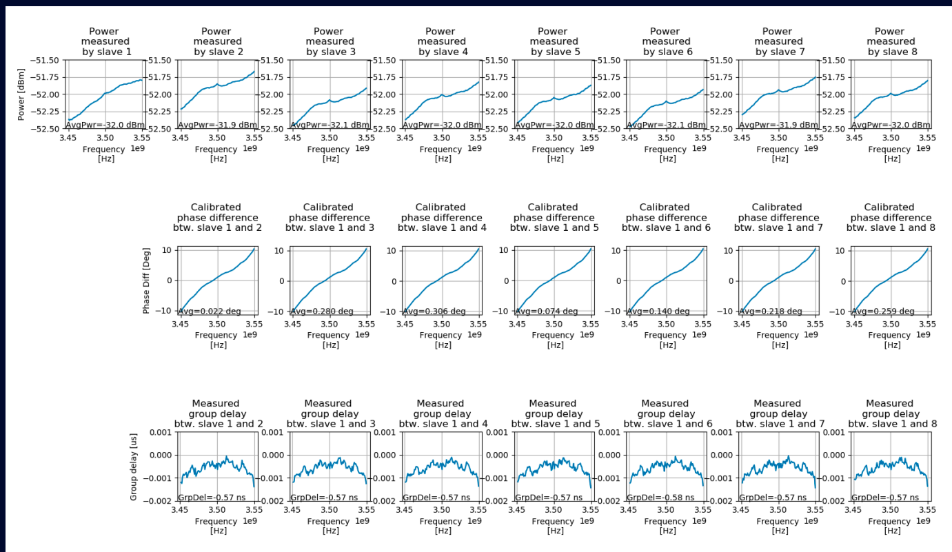
1台のR&S®NRQ6マスターと8台のR&S®NRQ6スレーブによる、マルチチャネルの位相差測定のサンプル結果。 マスターのR&S®NRQ6は、TRG、CLK、LO信号の分配のみに使用されます。
