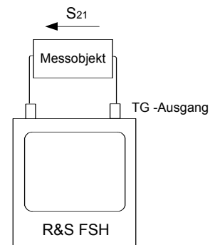
Bild 4: Messaufbau für eine Transmissionsmessung mit dem R&S FSH
