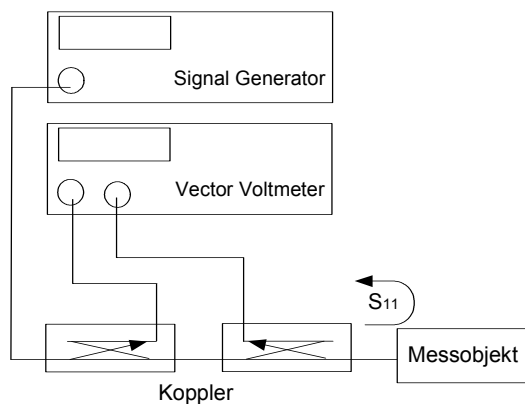
Bild 1: Traditioneller Messaufbau für eine Reflexionsmessung mit einem Vektor-Voltmeter
