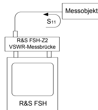
Bild 2: Messaufbau für eine Reflexionsmessung mit dem R&S FSH
