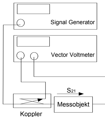
Bild 3: Traditioneller Messaufbau für eine Transmissionsmessung mit einem Vektor-Voltmeter
