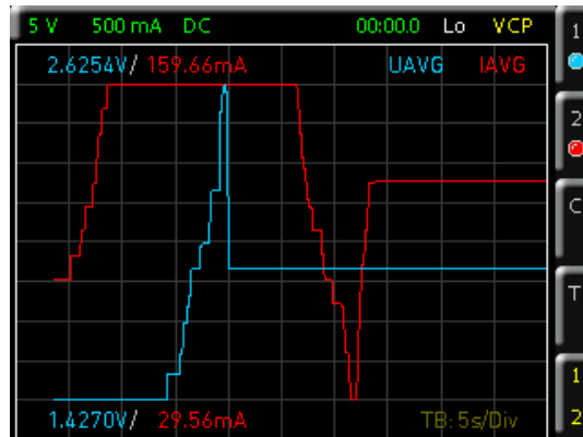
Abb. 6.8: Trendchart Modus
