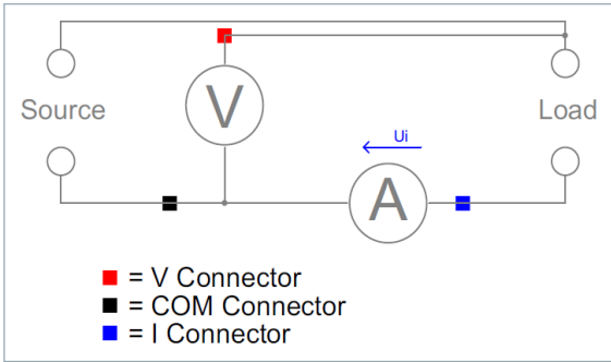
Abb. 4.7: Stromrichtige Messung
