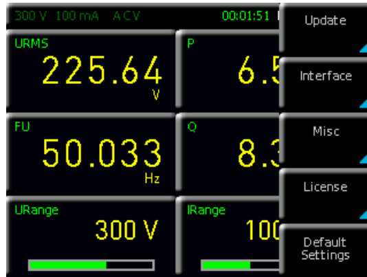
Abb. 9.1: Setup-Menü
