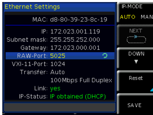
Abb. 10.11: Ethernet Einstellungen
