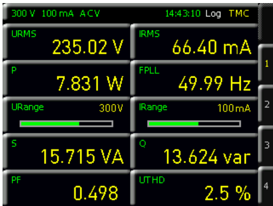
Abb. 6.1: Messwertanzeige R&S®HMC8015
