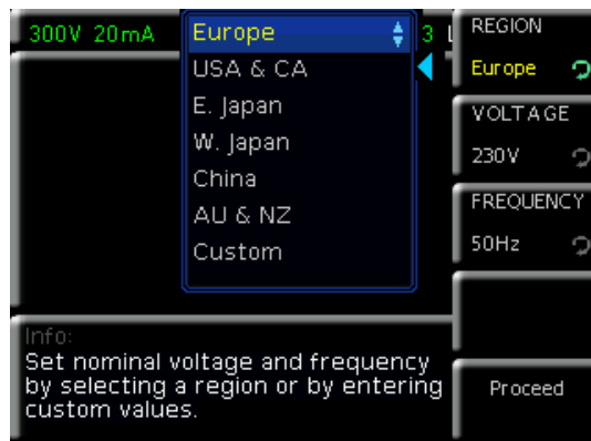
Abb. 6.13: Einstellungsmenü EN 50564
