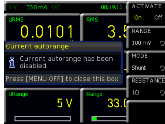
Abb. 4.10: Sensor-Menü
