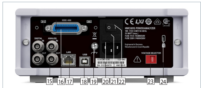
Abb. 2.2: Geräterückseite R&S®HMC8015
