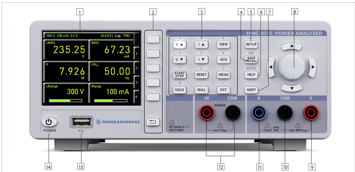
Abb. 2.1: Gerätevorderseite R&S®HMC8015
