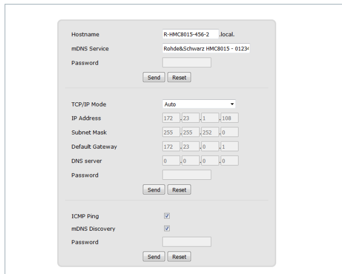
Abb. 10.13: Ethernet-Einstellungen
