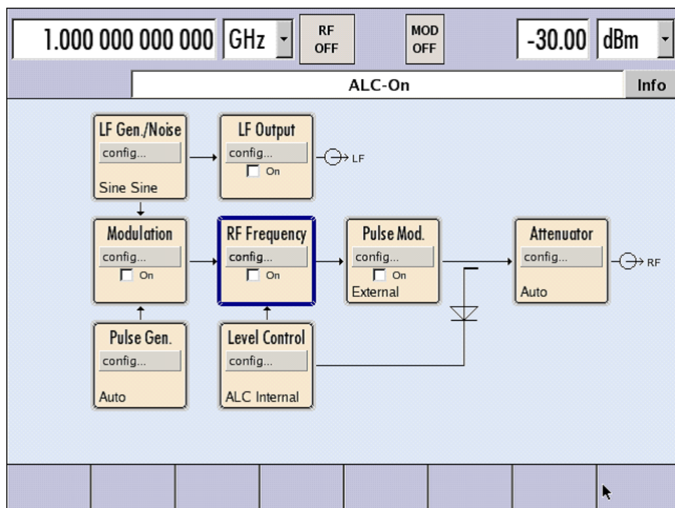
図 4-1: すべての機能を装備した R&S SMF のブロック・ダイアグラム
