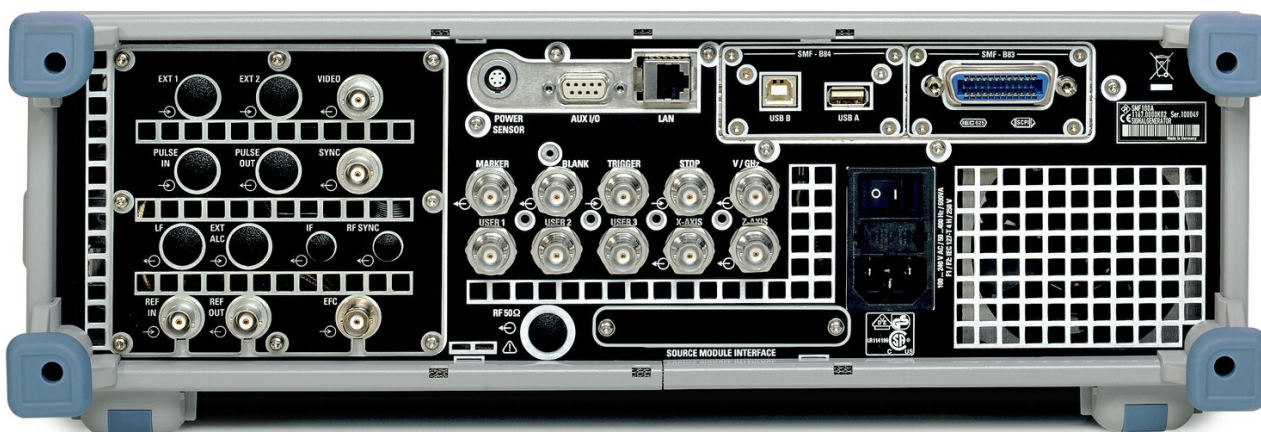
図 2-2: リア・パネル
