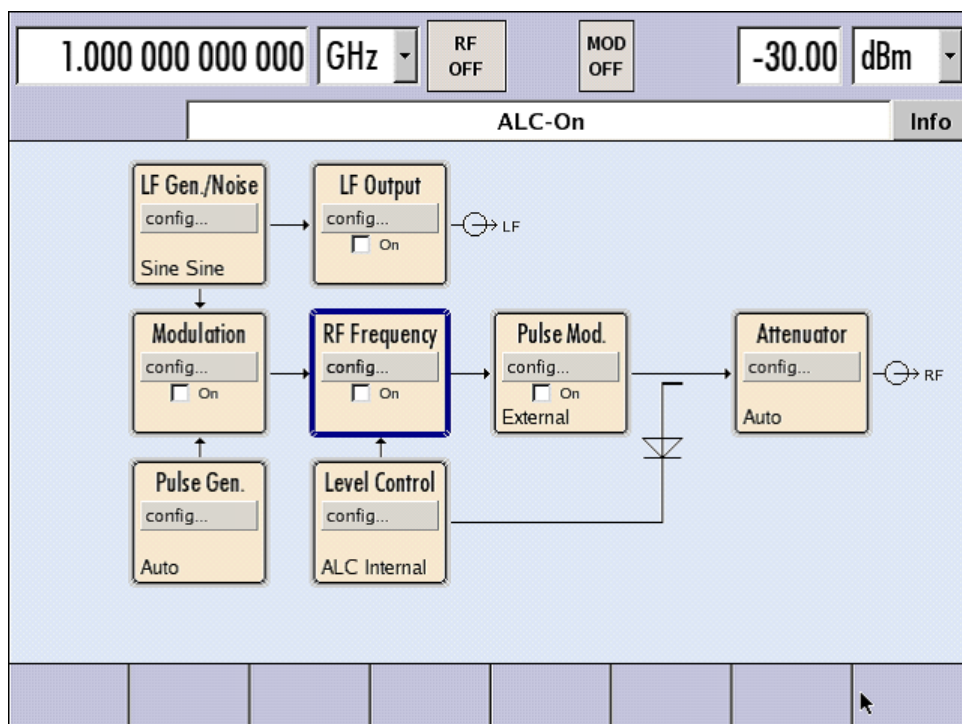
図 3-1: すべての機能を装備した R&S SMF のブロック・ダイアグラム
