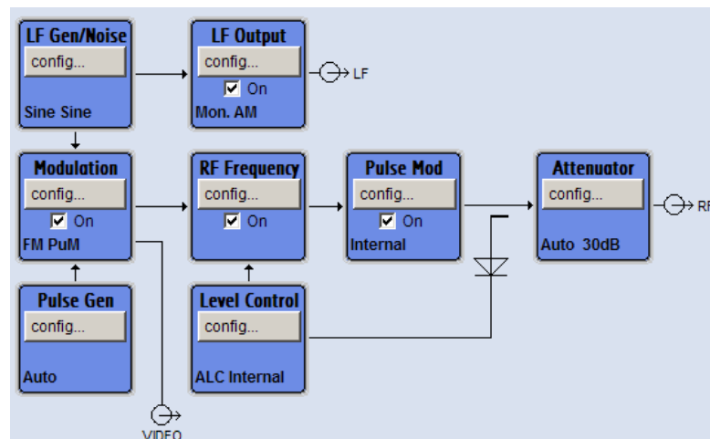
図 4-2: R&S SMF のブロック・ダイアグラム
