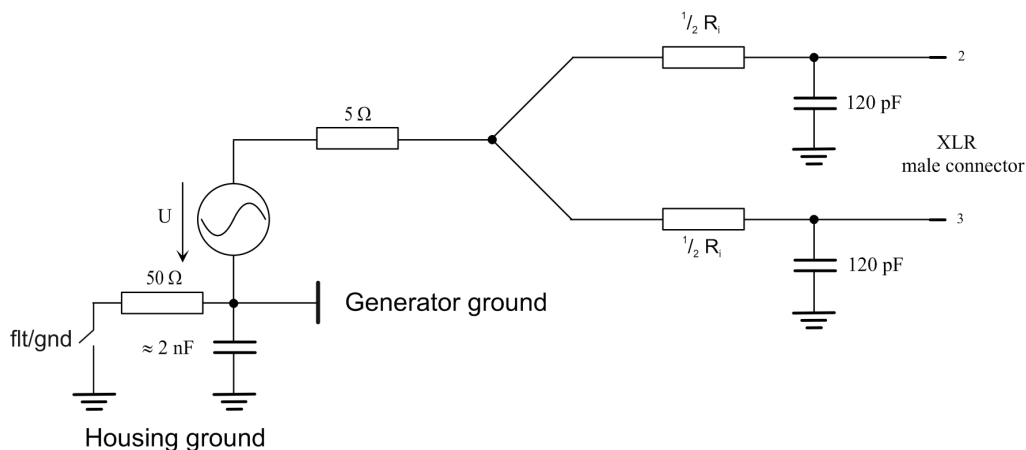
Bild 5-10: Ausgang mit Gleichtaktsignal
