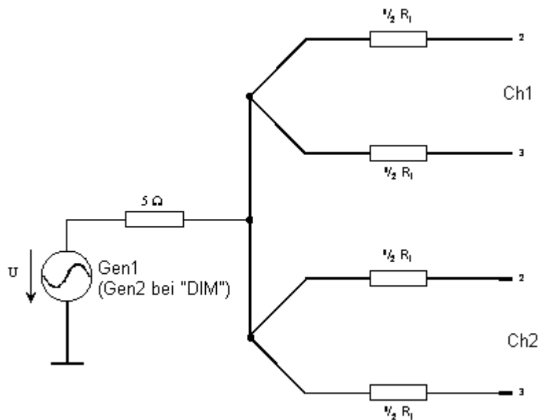
Bild 5-12: Channel 2 = 1
