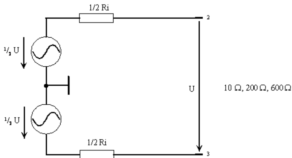
Bild 5-6: Channel = 1 oder 2
