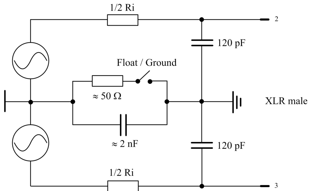
Bild 5-5: Symmetrischer Ausgang
