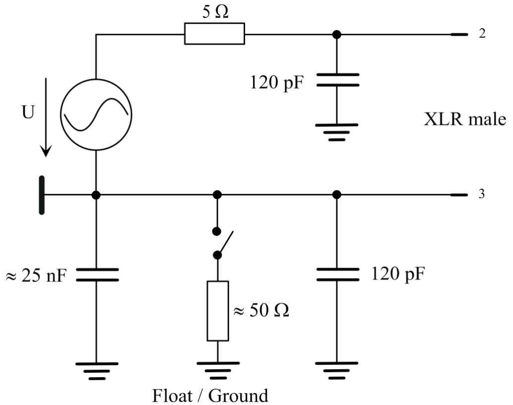
Bild 5-2: Unsymmetrischer Ausgang
