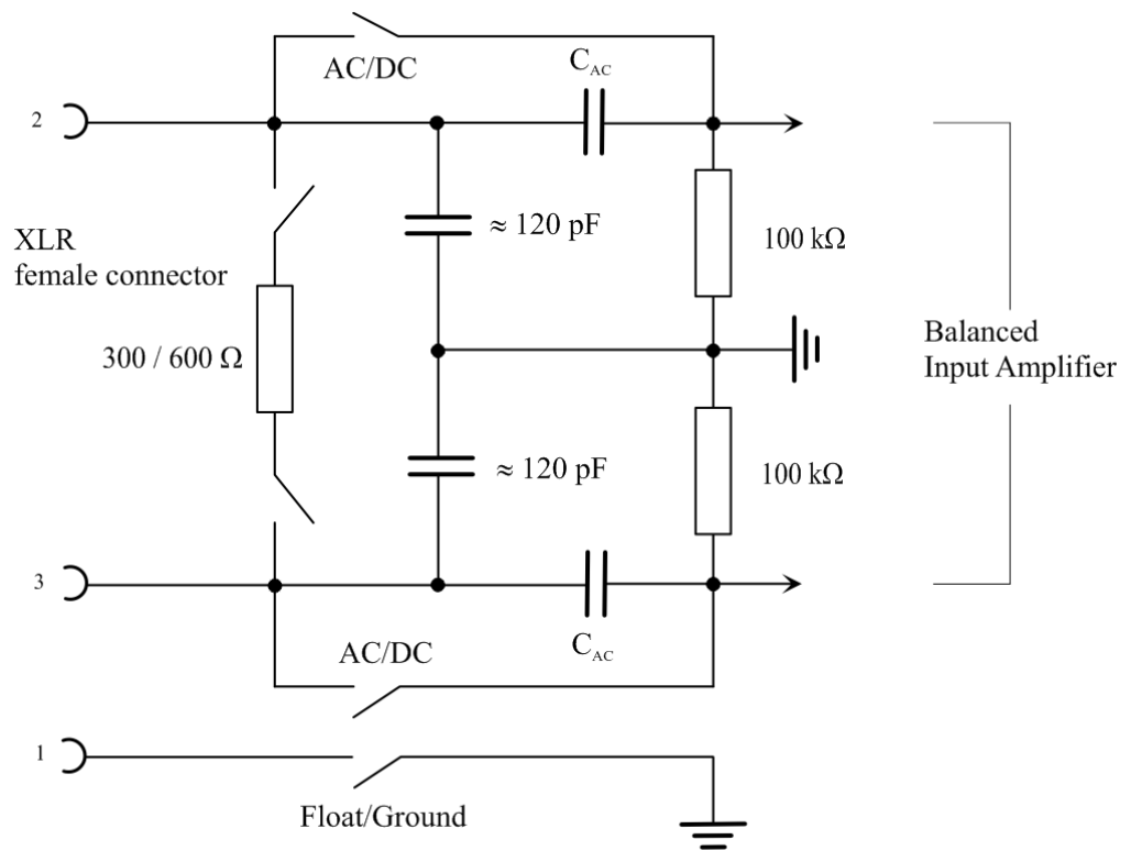
Bild 5-14: Symmetrischer Analyzer-Eingang
