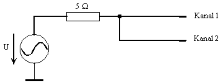
Bild 5-4: Channel = 2 = 1
