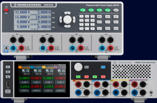
R&S®HMP4040 및 R&S®NGP804 4채널 파워 서플라이
