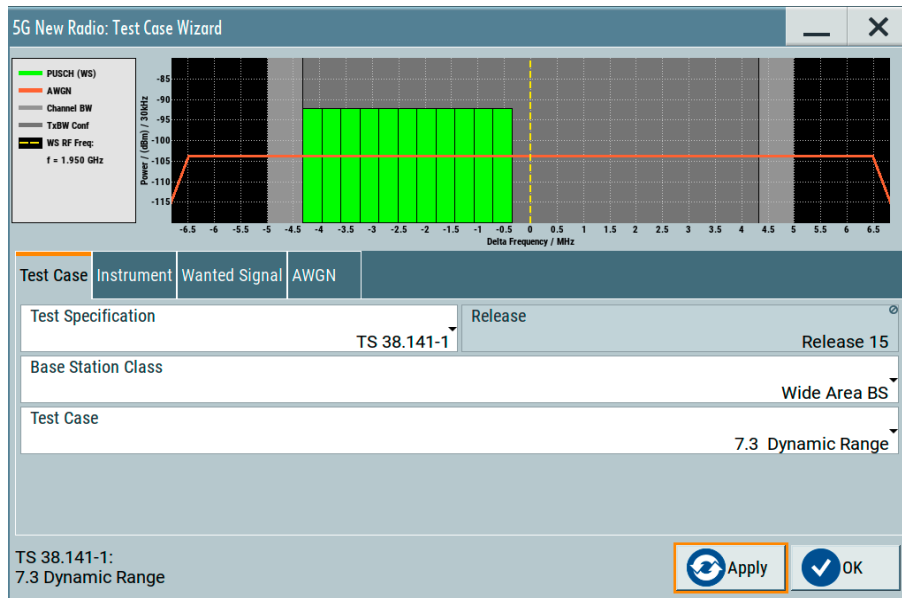
5G NR测试用例向导能够便捷灵巧地配置R&S®SMM100A,以根据3GPP TS 38.141进行基站收发机测试
