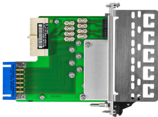
R&S®TS-PRIO3, rear I/O module for R&S®TS-PSM3
