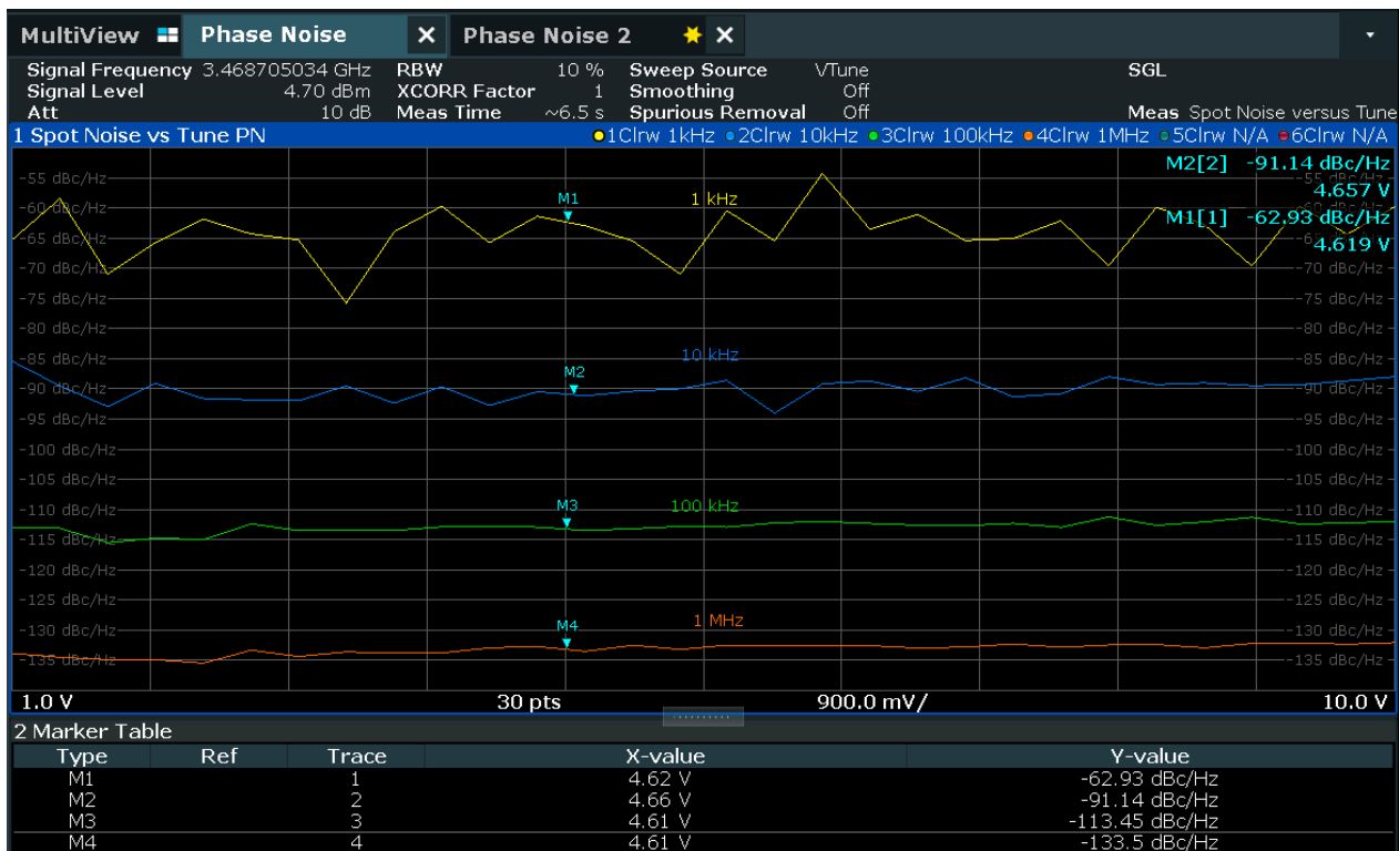
1 kHz、10 kHz、100 kHz、1 MHz 偏移频率下相对于调谐电压的 VCO 相位噪声
