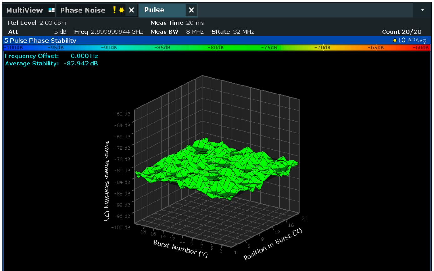
多个脉冲序列(脉冲串)的脉冲相位稳定性 3D 图
