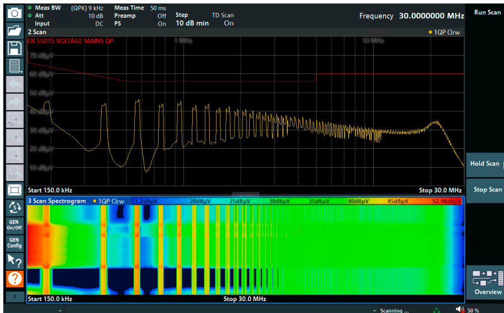
分析LED灯在亮度变化时的发射。使用准峰值检波器完成测量。
