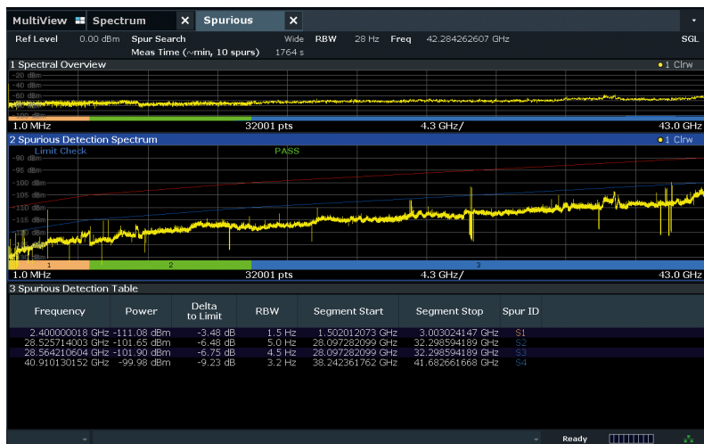
スプリアス測定の結果画面
