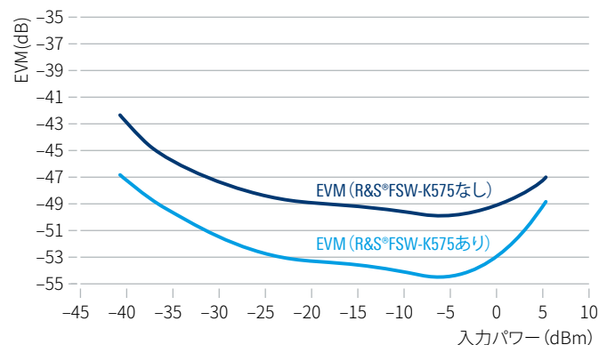
6.905 GHz、320 MHzのWi-Fi® IEEE 802.11be信号入力時の残留EVM対信号パワー (変調次数4096QAM)
