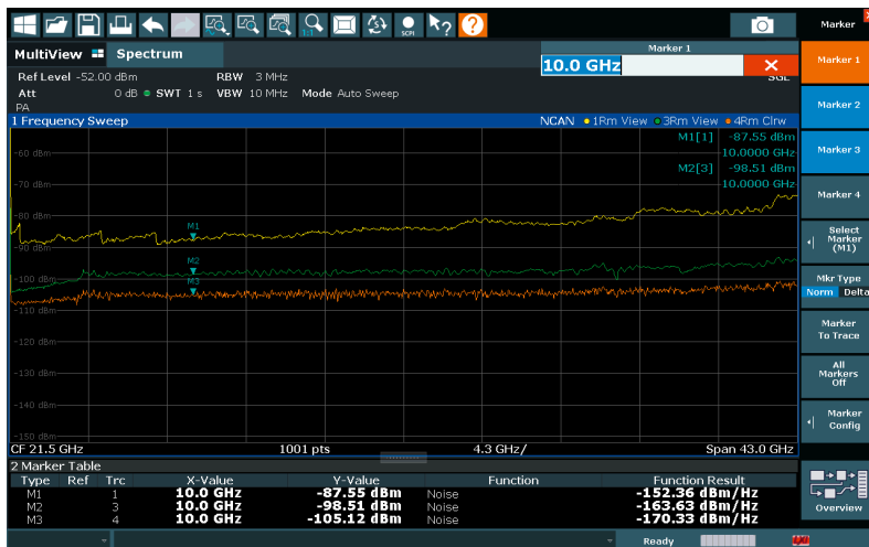
プリアンプおよびノイズキャンセルをオン/オフにしたR&S®FSW43の表示平均雑音レベル (DANL)
