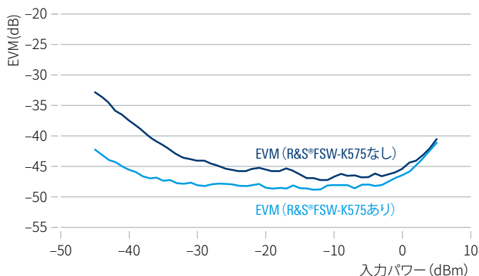
28 GHzで帯域幅100 MHzの5G NRダウンリンク信号の信号パワー全体の残留EVM
