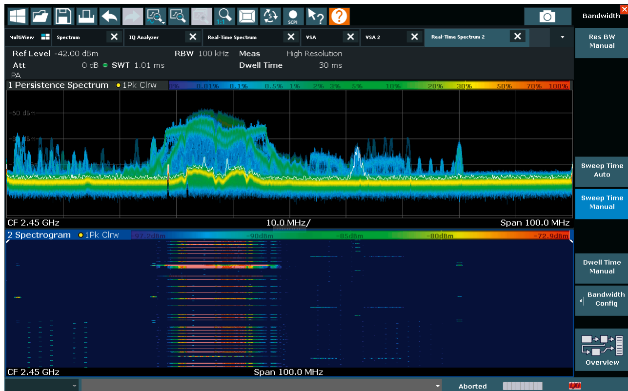
2.4 GHzでのISMバンドのリアルタイムスペクトラム
