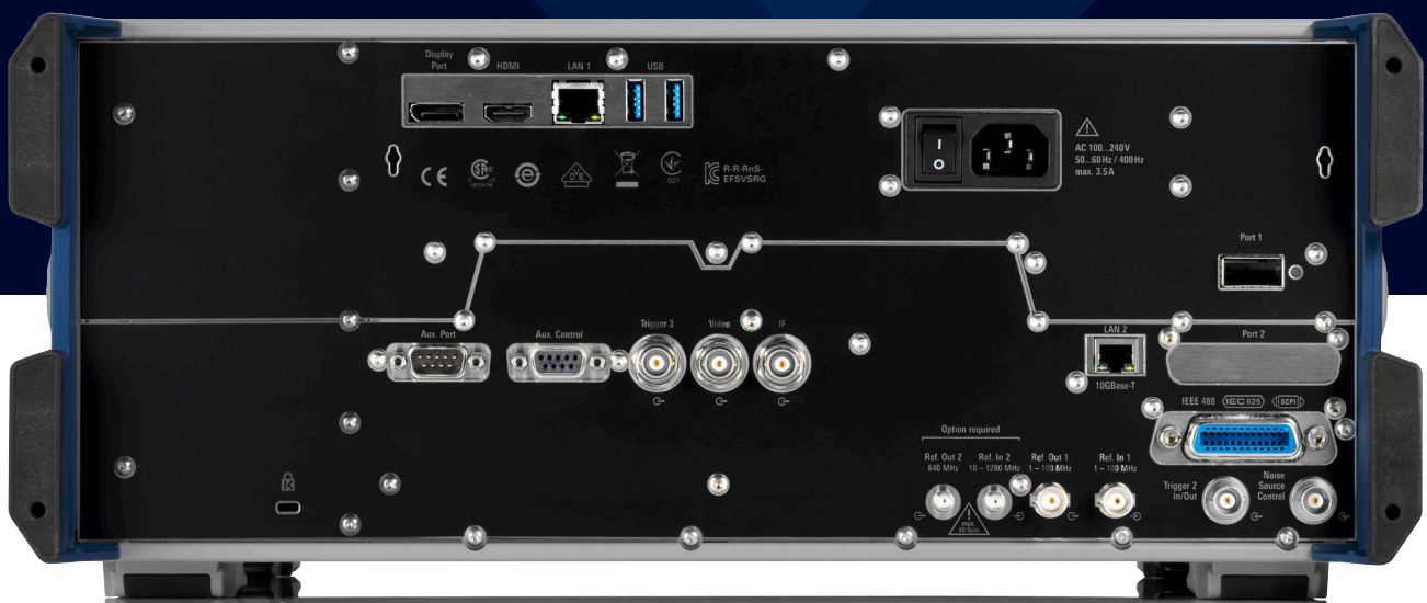
R&S®FSVA3000 后视图。
