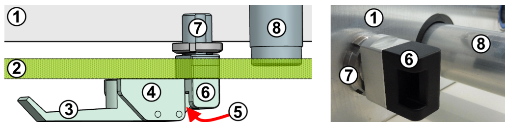
आंकड़े 7-2: ओवर-सेंटर कम्प्रेसन-लैच मैकेनिज्म (बाएं), और विवरण चित्र (दाएं) का क्रॉस-अनुभागीय शीर्ष दृश्य
