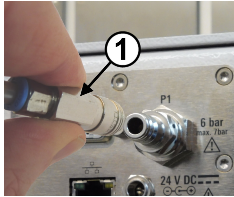
आंकड़े 6-5: संपीड़ित-हवा की सप्लाई को जोड़ना
