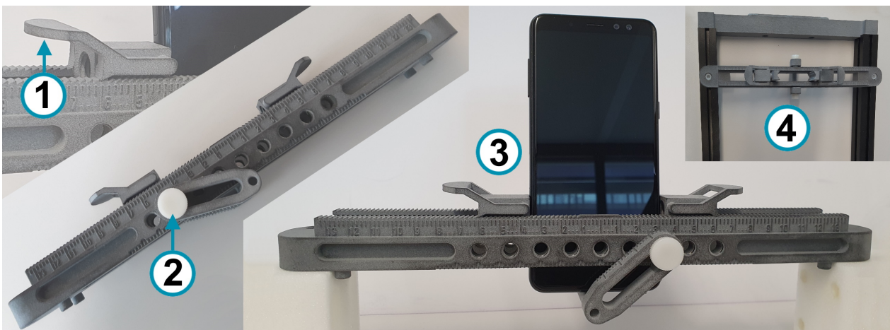
รูป 7-10: R&S CMQ-B714A ตัวเลือก "DUT Clamp 1", เลขคำสั่งซื้อ 1537.6255.02
