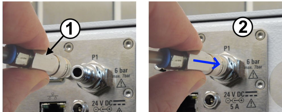
圖 6-5: 連接壓縮空氣供給系統
