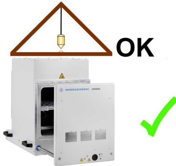
圖 6-1: 屏蔽箱的水平位置
