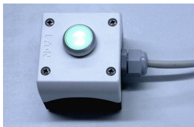
图 7-3: 按钮上的绿色指示灯指示屏蔽箱门已关闭
