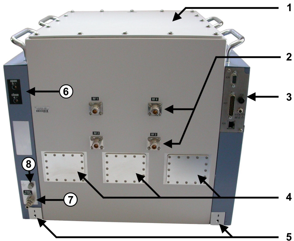
图 4-3: 屏蔽箱后视图
