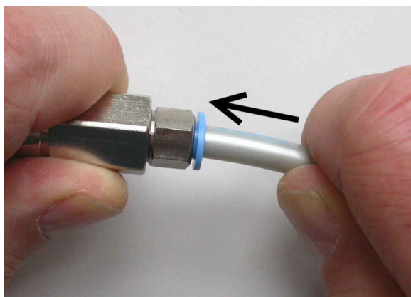
图 6-7: 装配推挽式适配器（左）和 6 mm 挠性管（右）
