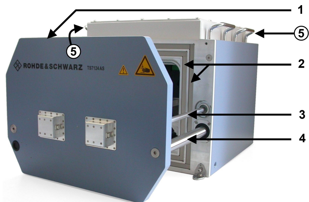
图 4-1: 门打开的屏蔽箱前视图
