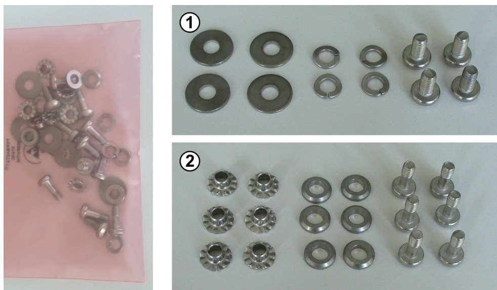
图 6-5: 一套梅花螺丝和垫圈，包含在机架安装套件中
