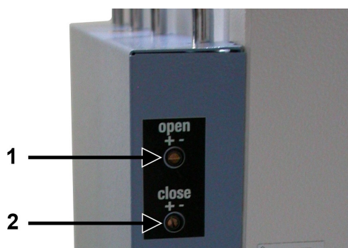
图 6-12: 用于调整气动系统的螺钉
